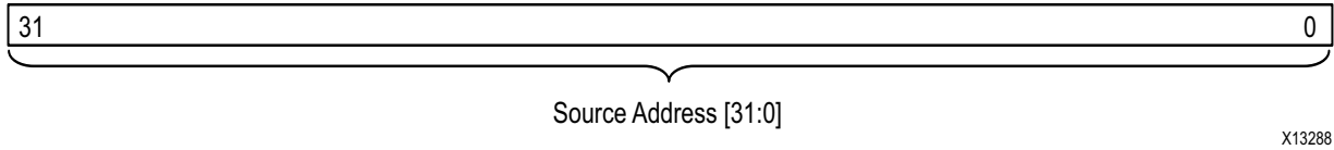
Figure 2-8: SA Register
