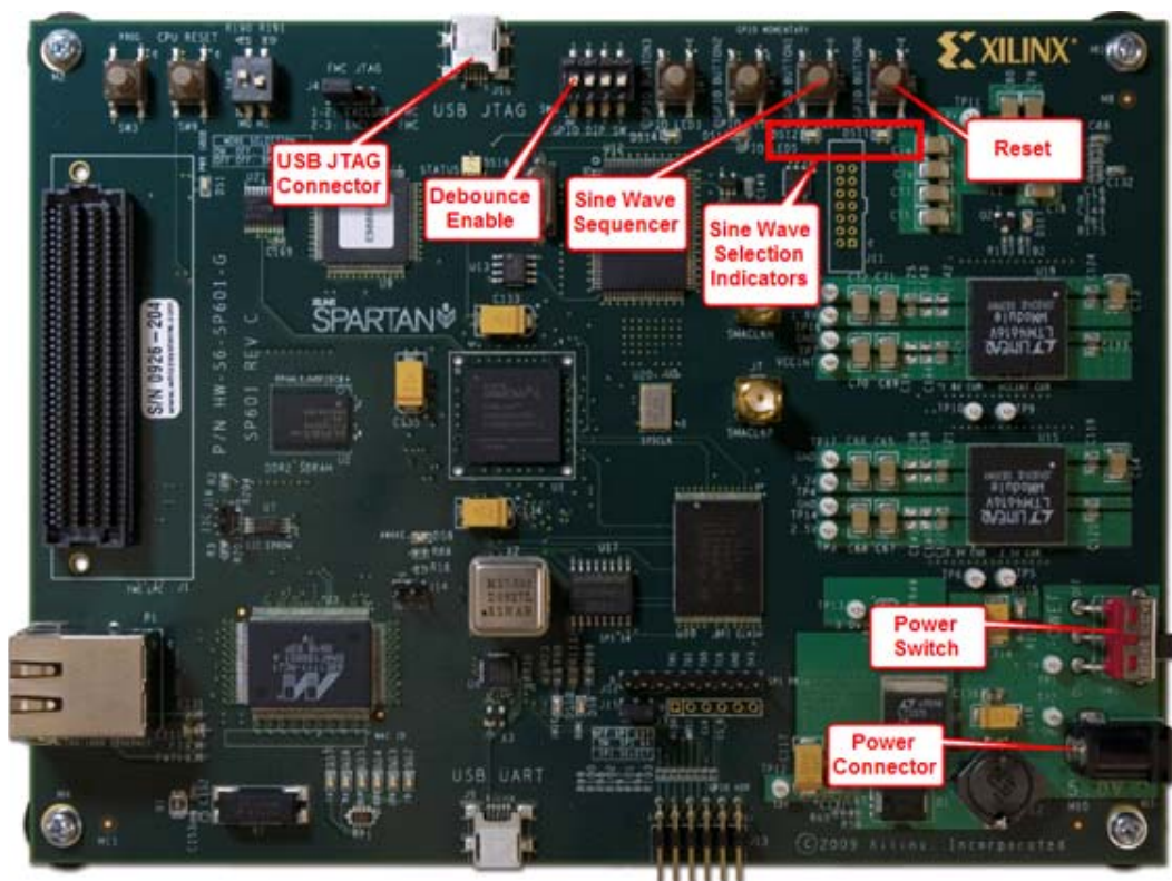
図 1 : SP601 ボード
